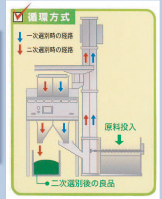
＜循環方式垂直バケット＞
