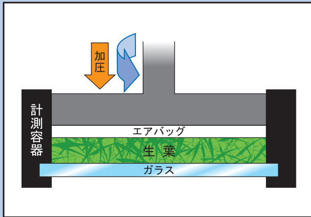
●生葉計測室構造●
